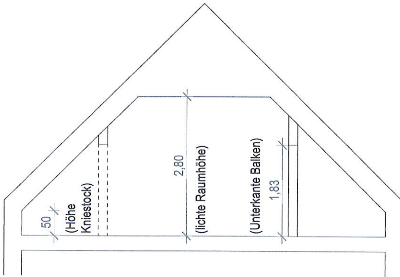
vereinfachter Schnitt der Höhen im Dachgeschoss
