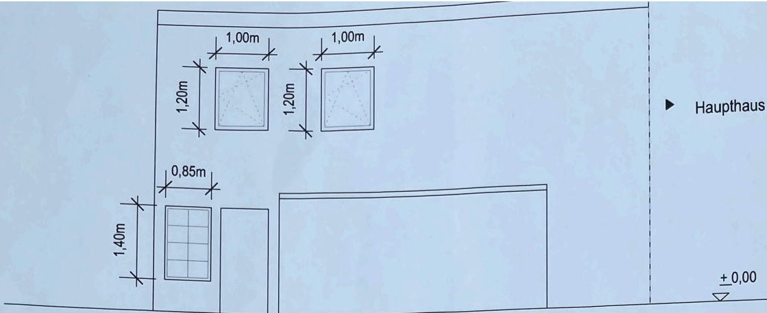
Ansicht West M 1:100
