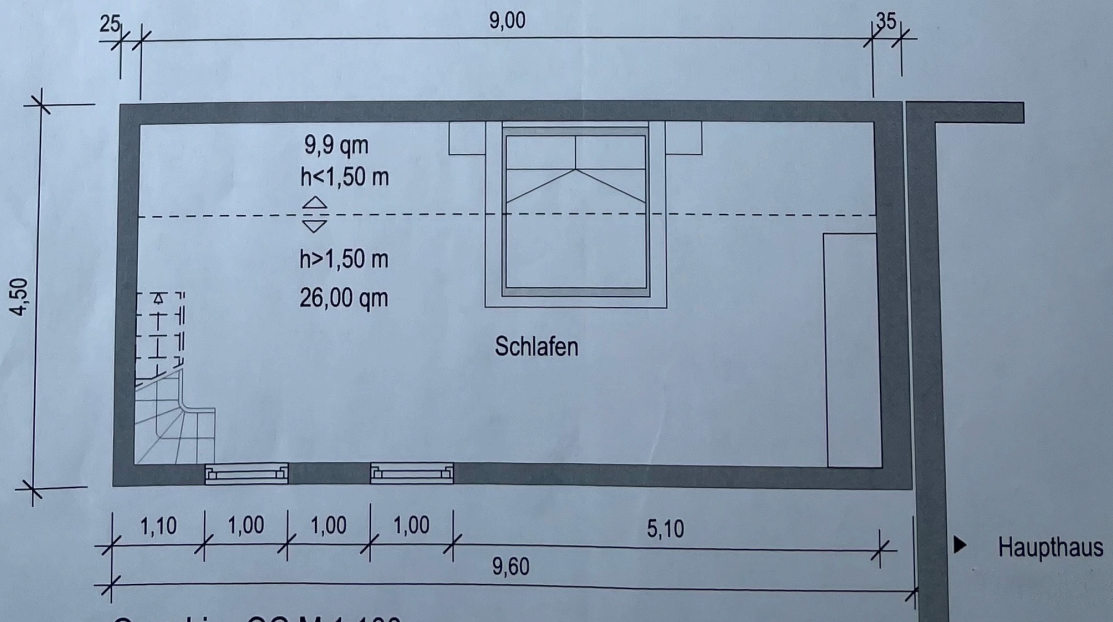
Grundriss OG M 1:100
